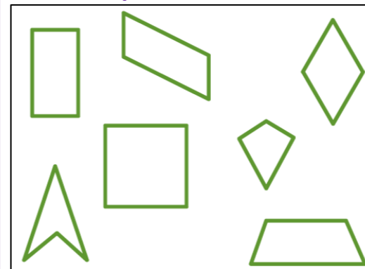
Quadrilaterals
