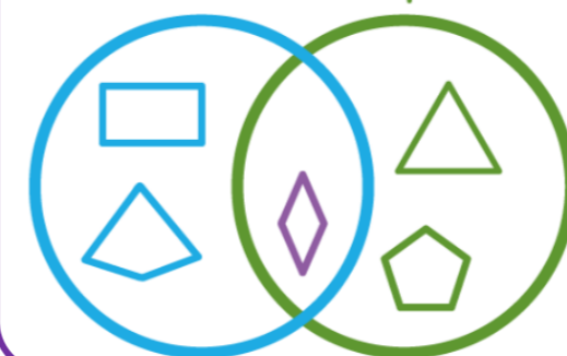
Quadrilaterals
